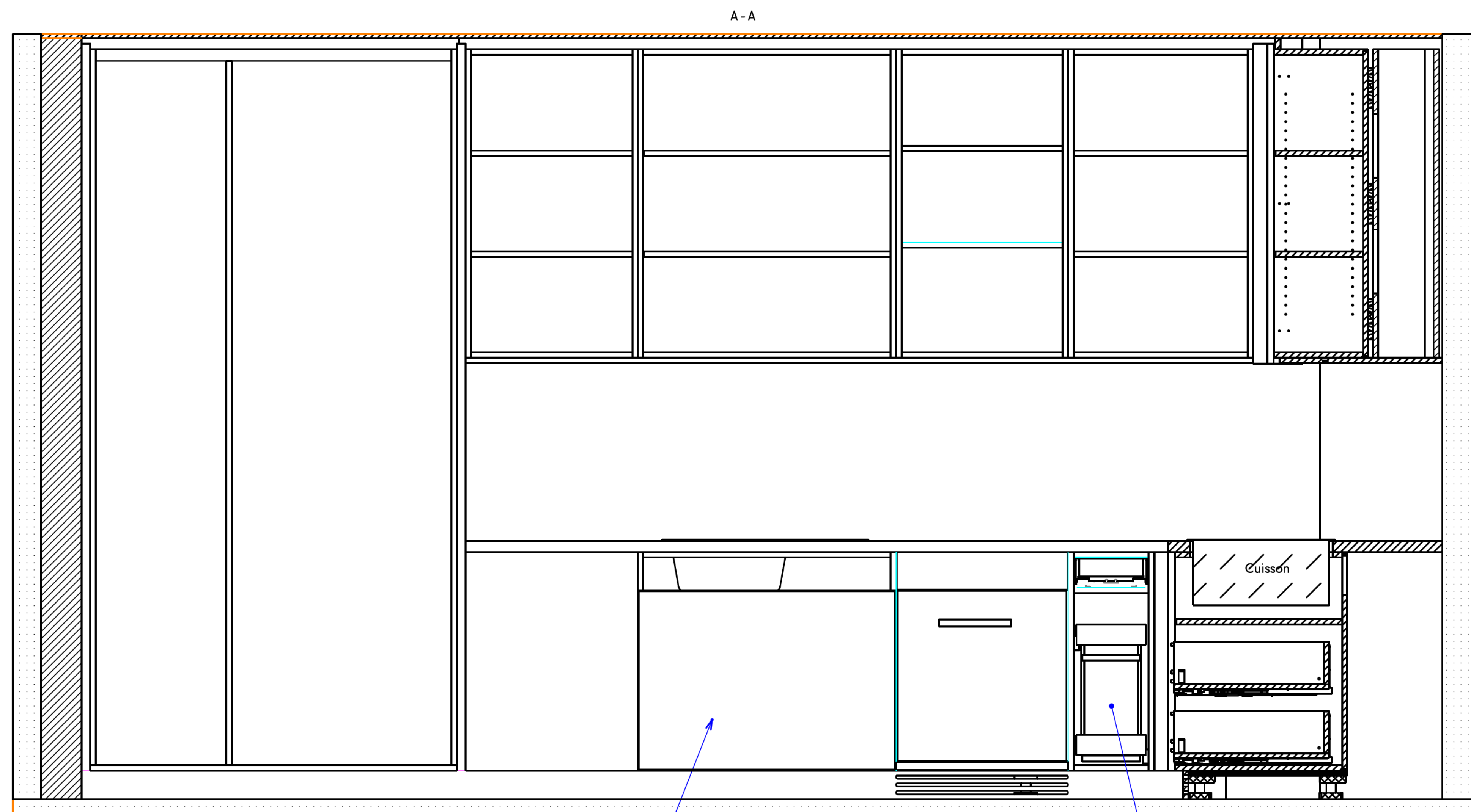
Tiroir légrabox ht. K Ref Foussier : 241401 Equipement poubelle : Ref LMC : SET5169GRTA BAC5060GRA BAC5051GRA Tiroir à l'anglaise Légrabox ht. M Ref Foussier : 280952
